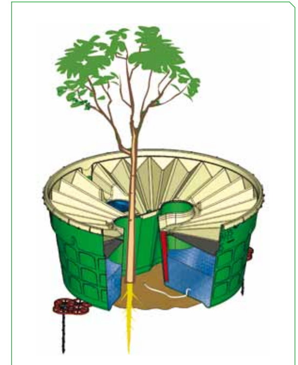
QUERSCHNITT DER WATERBOXX FOTO: © GROASIS
